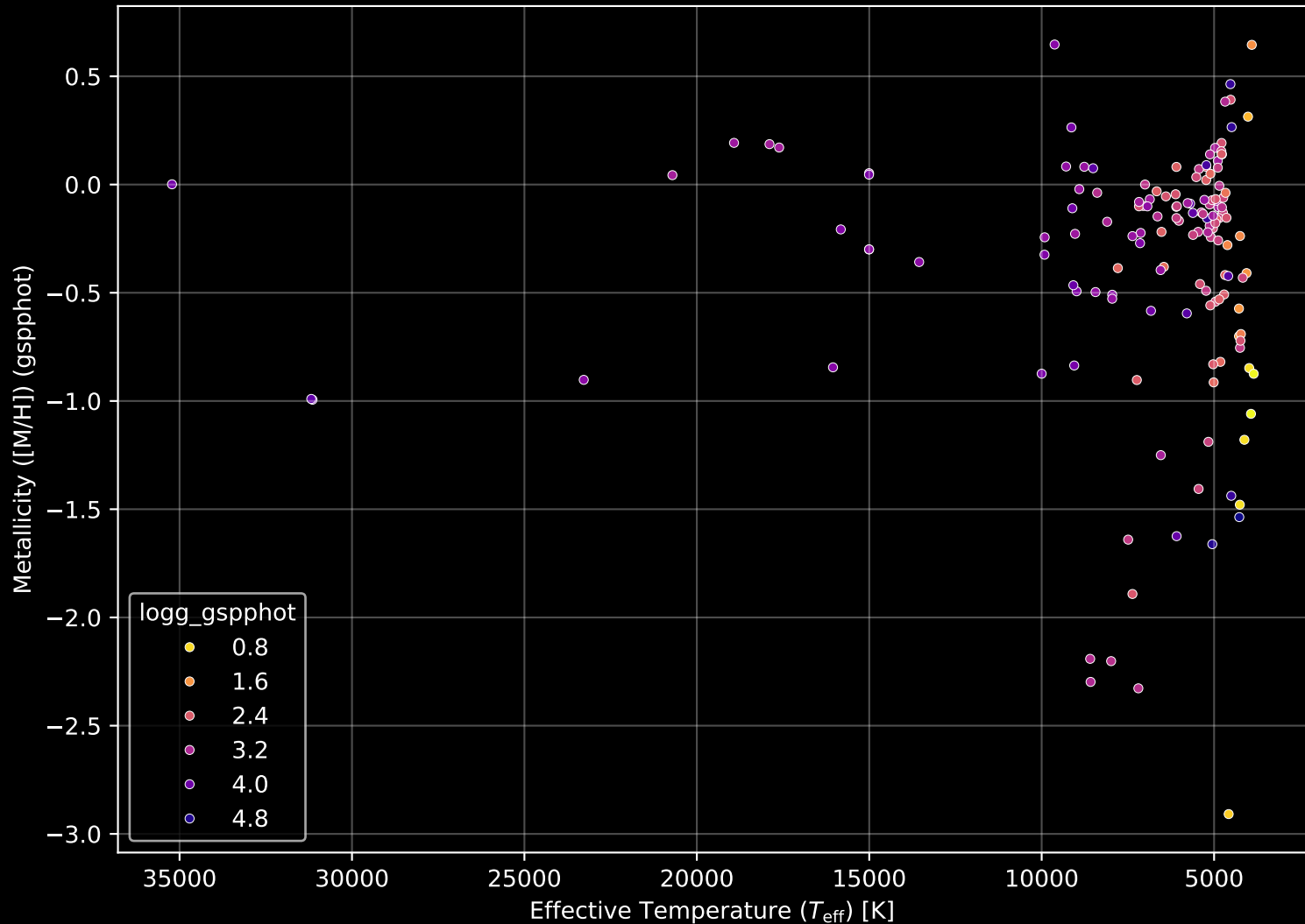
APOGEE DR17 Field: [285+00] Stellar Population Parameters (n= 148)
